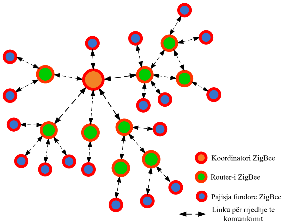
Figura 4.5. Topologjia Hibride
