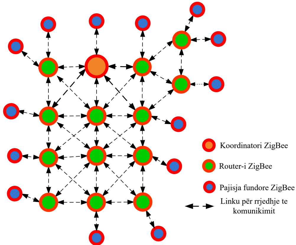
Figura 4.4. Topologjia mesh
