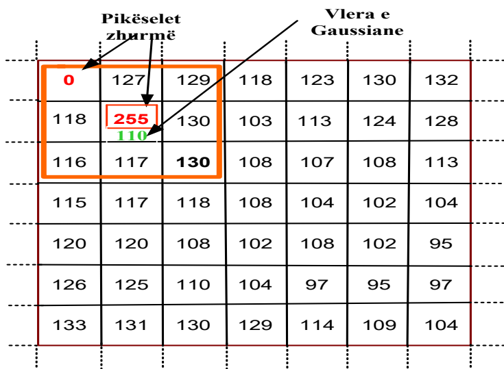
Figura 6.6. Parimi i punës së filtrit të Gausit në matricën e pikseleve të imazhit
