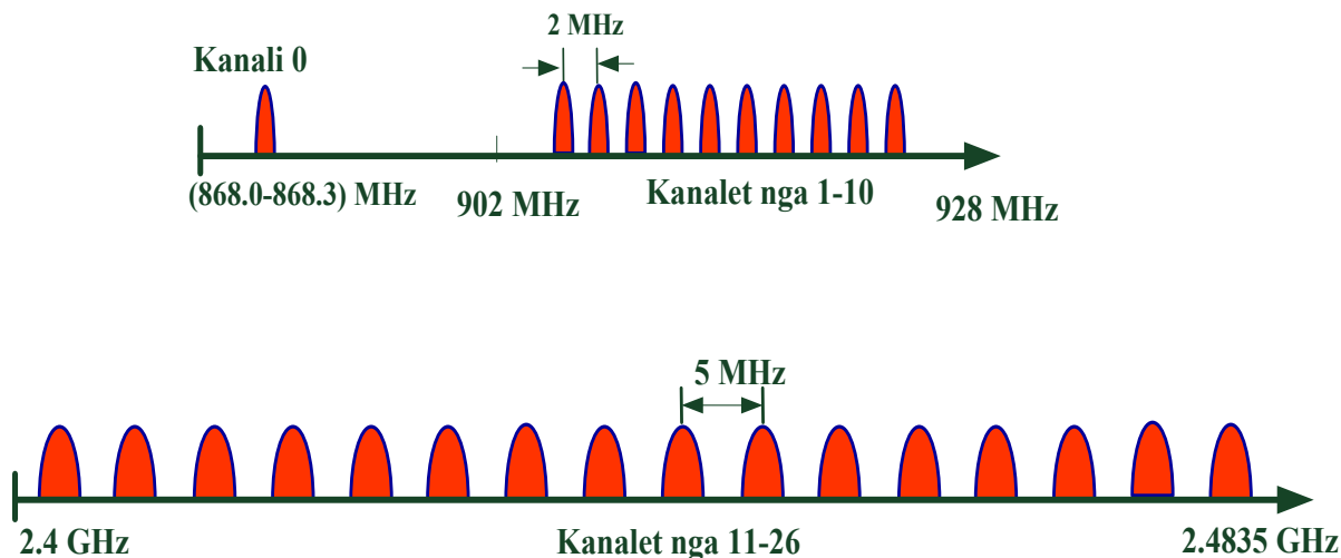
Figura 4.1. Brezët frekuencore operuese të standardit 802.15.4
