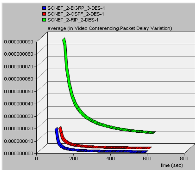
Figura 5.18. Luhatjet e vonesës së paketës për rastin e video aplikimeve
